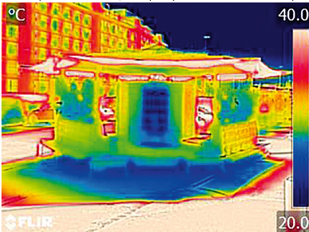
Le pavillon installé en juillet 2021 sur la place Python à Fribourg. Diamètre de la toiture avec le prolongement des toiles d'ombrage: 10 m, hauteur entre le plancher et la toiture: 2,5 m, hauteur maximale : 3,8 m. Sa structure modulaire permet de le démonter, le transporter puis le remonter sur un nouvel emplacement en ~1,5 jours.
