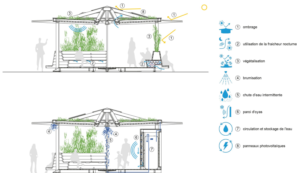
Coupes schématiques du pavillon et de ses dispositifs.
